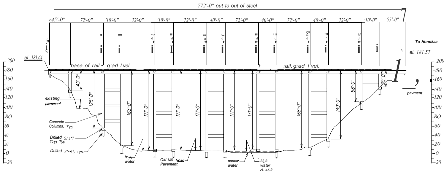
ELEVATION Scale: 1" = 40'-0"
